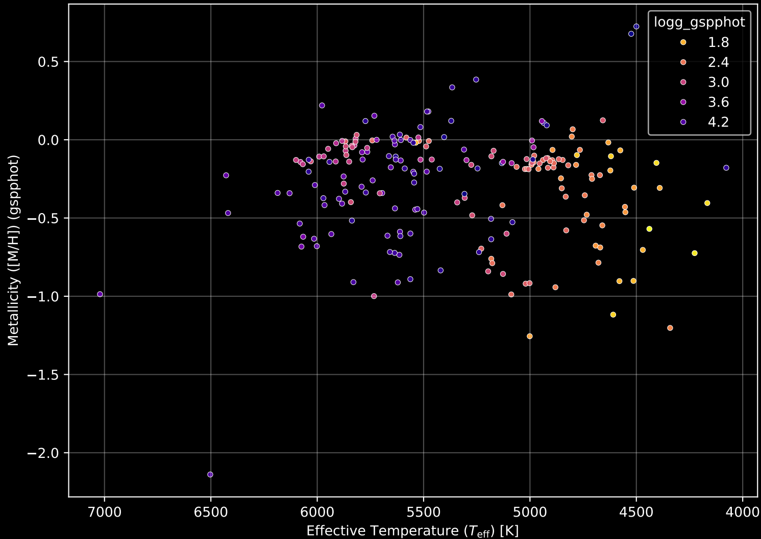
GALAH DR4 Field: [51] Stellar Population Parameters (n= 208)
