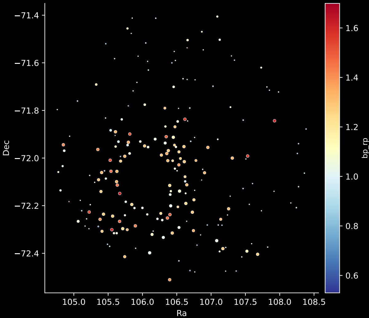
GALAH DR4 Field: [51] Stars: 208
