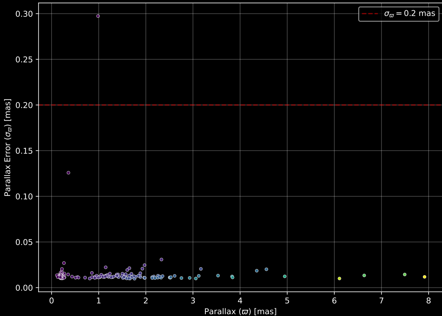
GALAH DR4 Field: [51] Parallax Quality (n= 208)
