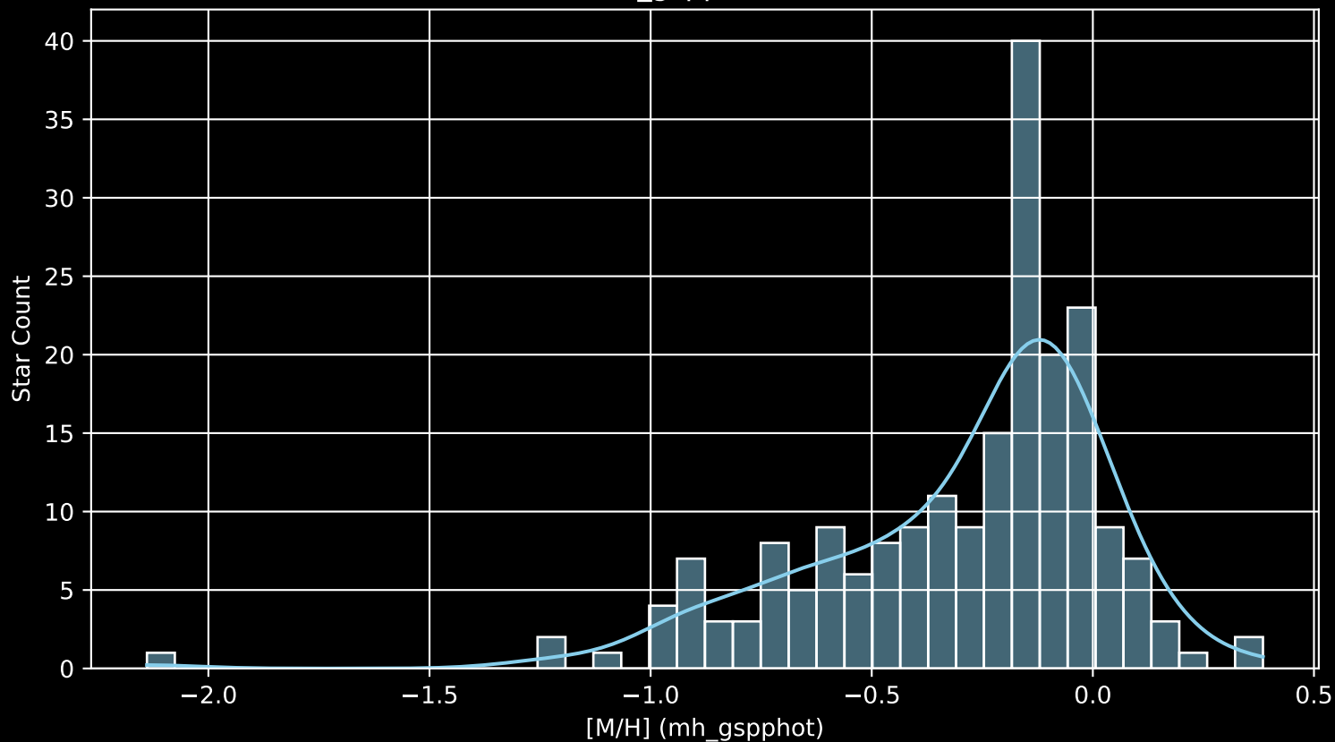
GALAH DR4 Field: [51] [M/H] (mh_gspphot) (n= 206)
